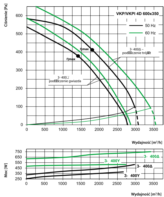
VKP 4D 600x350
