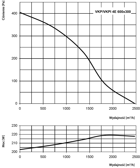
VKP 4E 600x300
