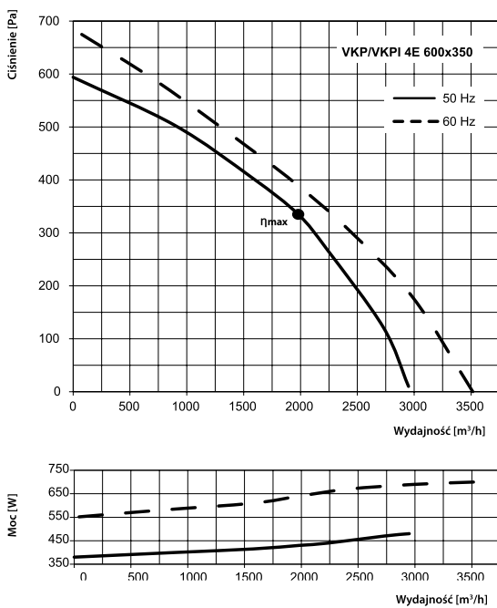
VKP 4E 600x350
