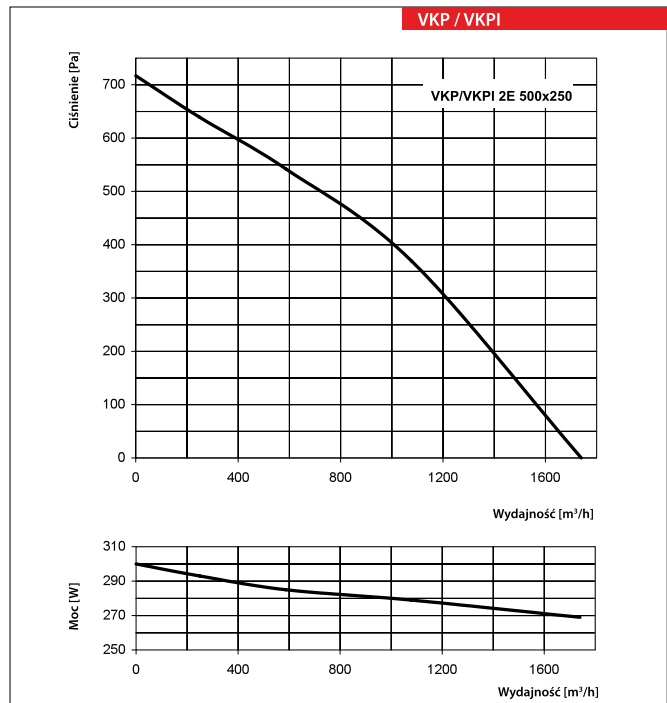
VKP 2E 500x250
