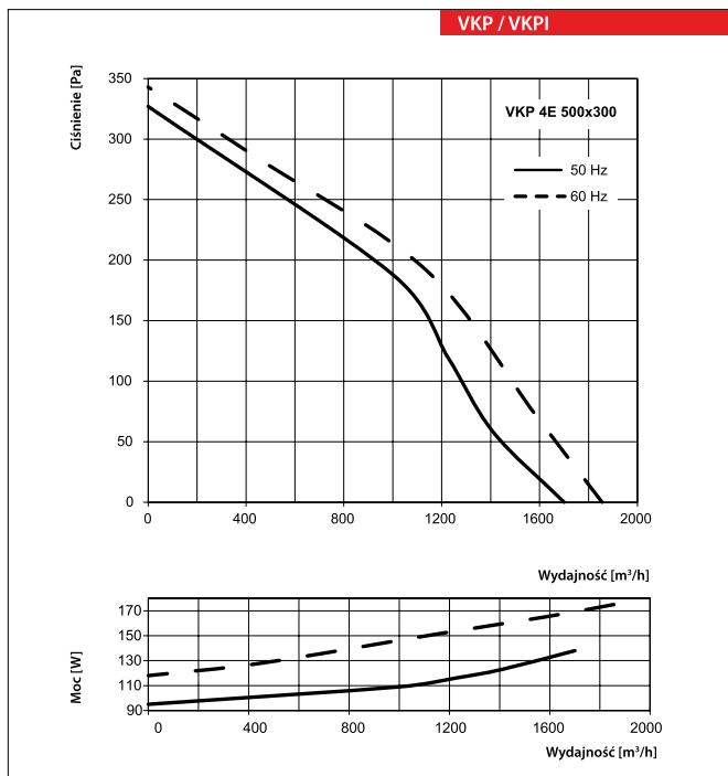
VKP 4E 500x300
