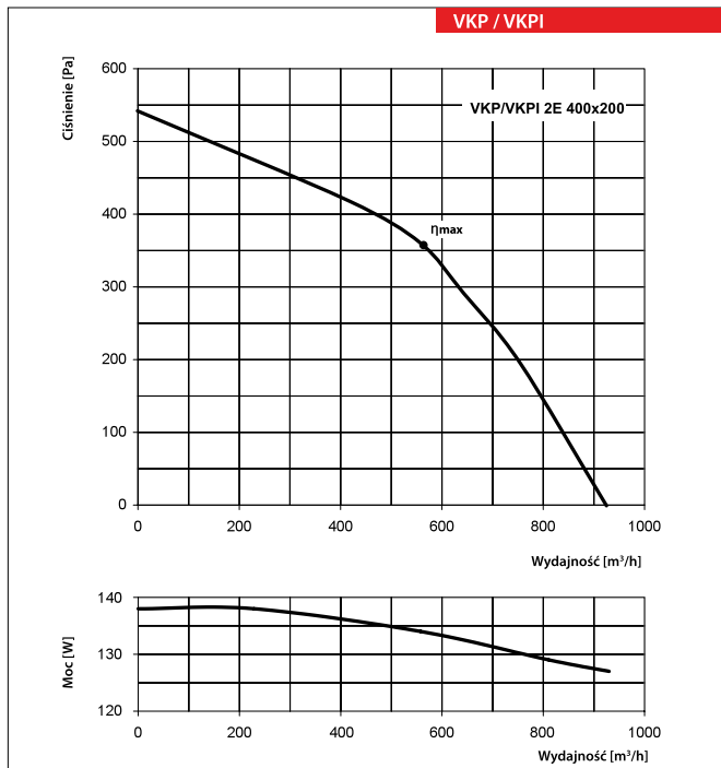
VKP 2E 400x200
